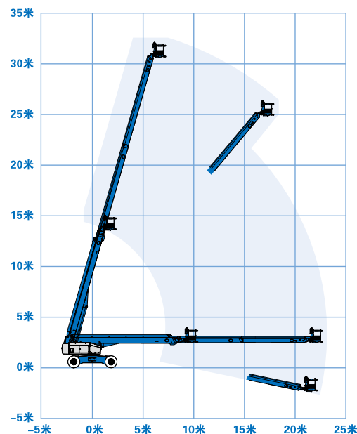
S™-100HD工作范围
