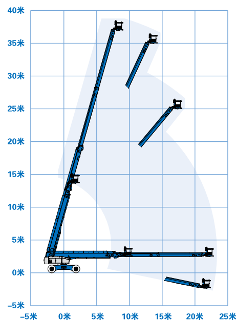
S™-120HD工作范围
