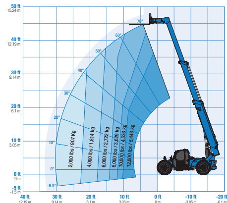
Diagrama de trabalho GTH-1244 sem estabilizadores
