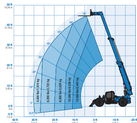
Diagrama de trabalho GTH-1244 com estabilizadores abaixados
