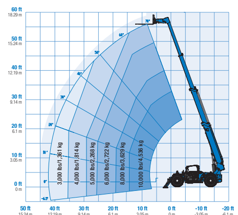
Diagrama de trabalho GTH-1056 com estabilizadores abaixados
