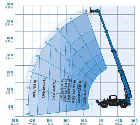
Diagrama de trabalho GTH-1056 com estabilizadores levantados
