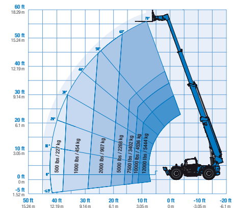
Diagrama de trabalho GTH-1256 with stabilizers up
