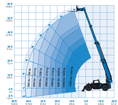
Diagrama de trabalho GTH-1256 with stabilizers down
