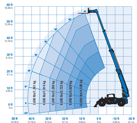
Diagrama de trabajo GTH-1056 with stabilizers down
