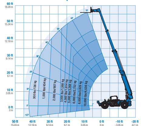
Diagrama de trabajo GTH-1056 with stabilizers up
