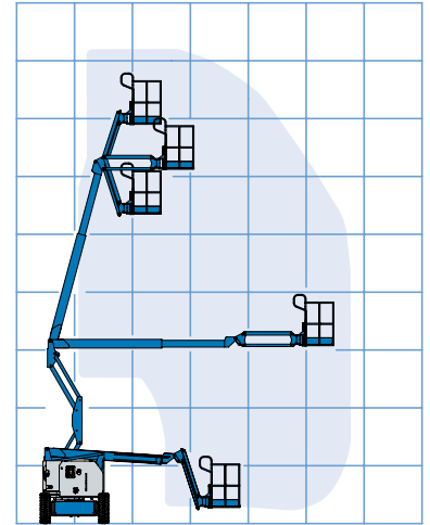
Z-34/22 IC工作范围
